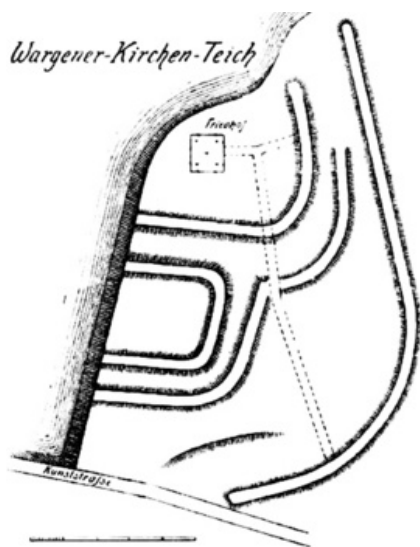
Vargių įtvirtinimų (pylimų) schema. Išlikę pylimai datuojami XIV a.
